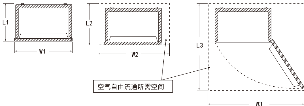
产品外形尺寸
