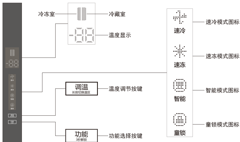
图示为BCD-520WBEPF2电脑控制面板及图解
