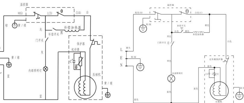
C*：电容C为可选件(根据压缩机选择)
